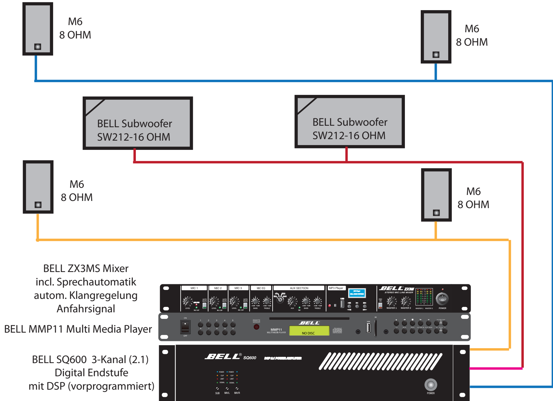
Beispiel: Musikanlage für Kinderfahrgeschäft (z.B. Dietz 10x10m)
